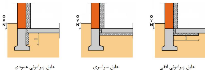
شکل پ ۱۱-۴ حالات مختلف عایق کاری حرارتی کف روی خاک به صورت کاهش یافته
