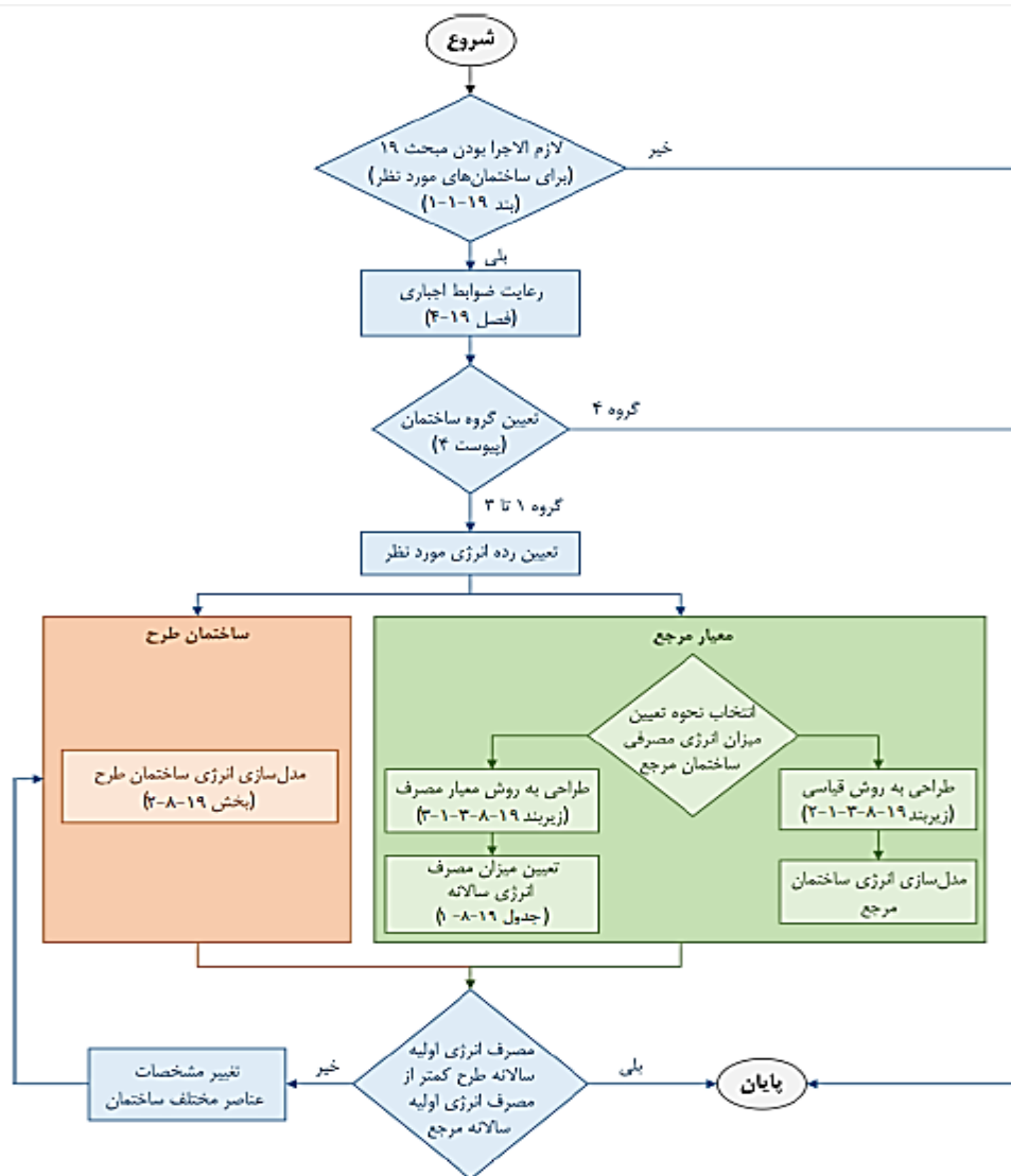
شکل ۸-۱۹-۱ نمودار گردش مراحل روش کارایی انرژی
