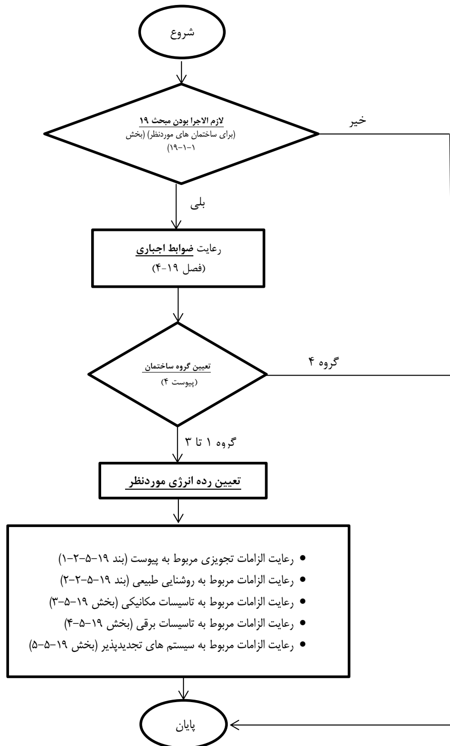
شکل ۱۹-۵-۱ نمودار گردش مراحل روش تجویزی
