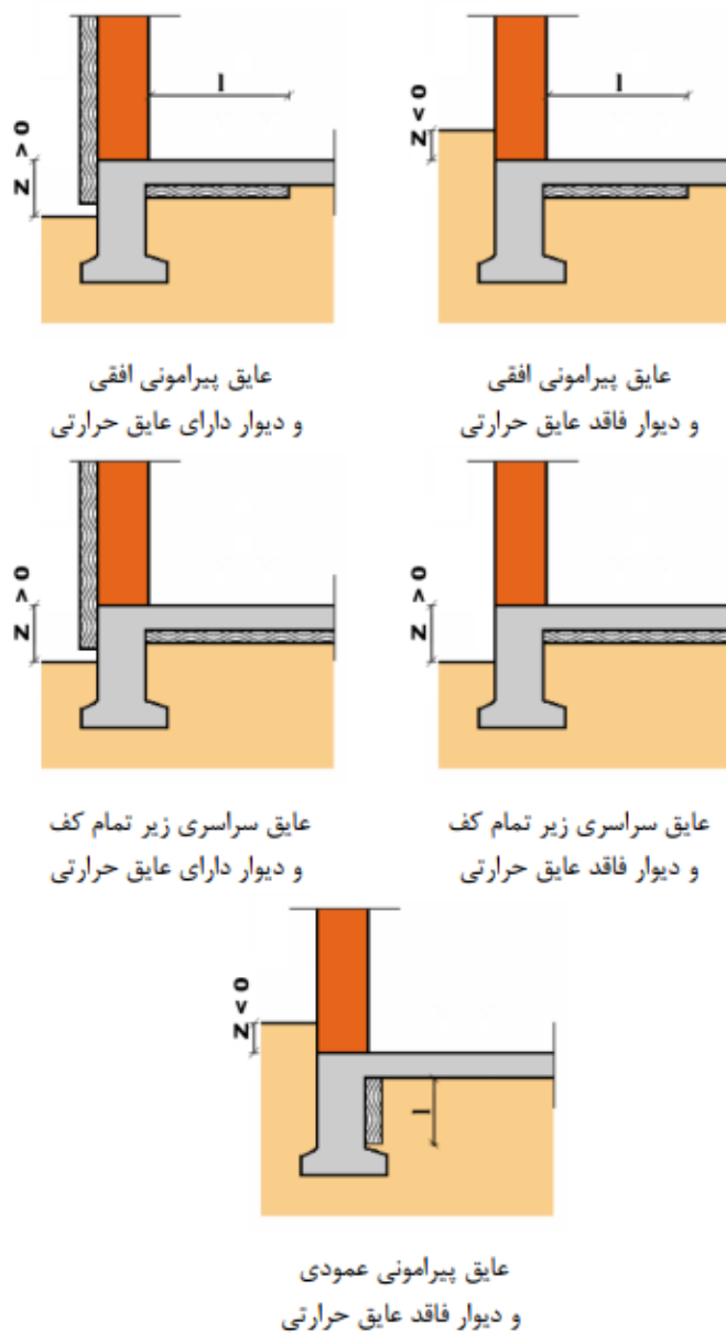
شکل پ ۱۱-۳ حالت‌های مختلف عایق‌کاری حرارتی کف روی خاک به صورت قطع شده در محل تلاقی دیوار و کف
