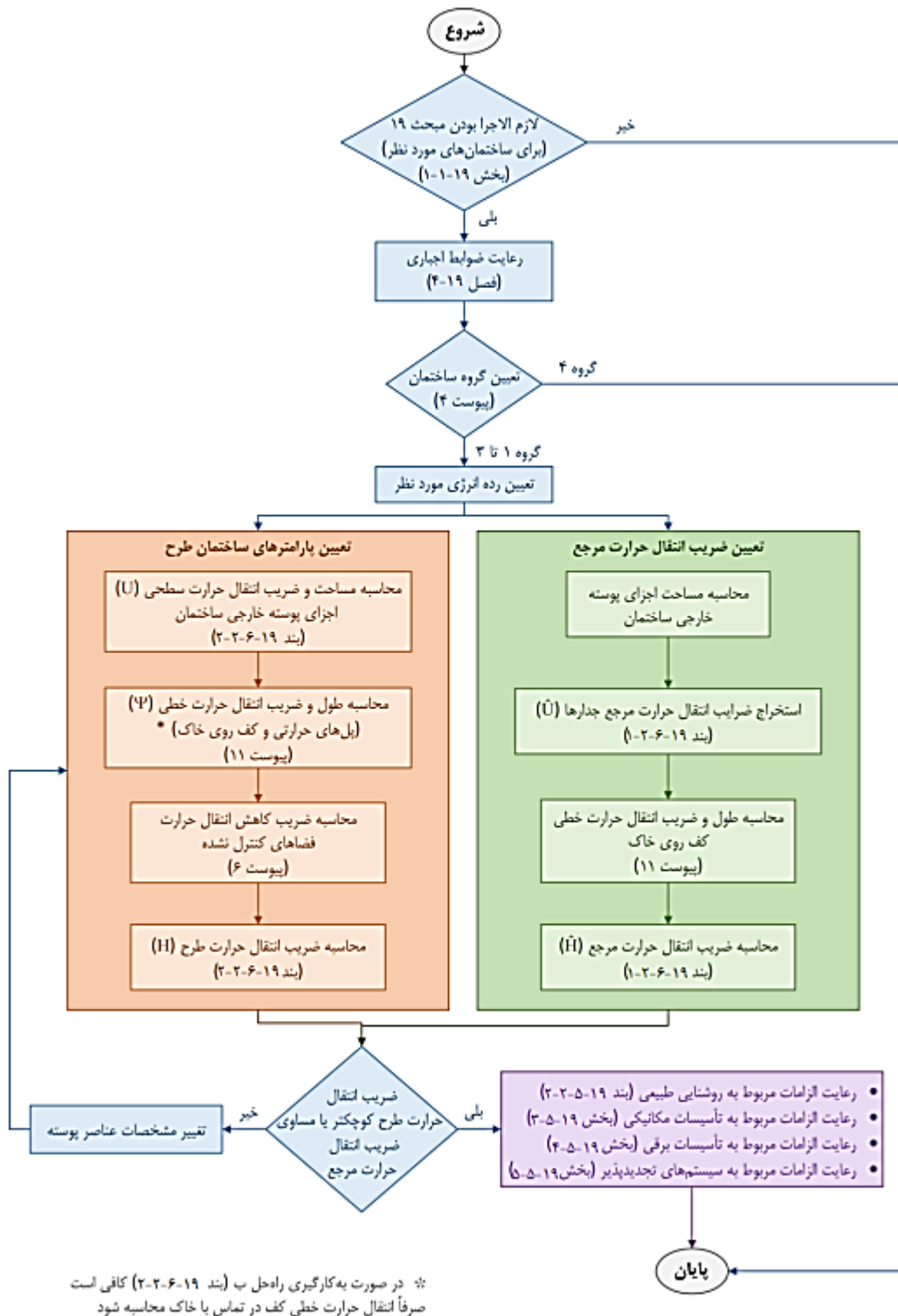
شکل ۱۹-۶-۱ نمودار گردش مراحل روش موازنه‌ای (کارکردی)
