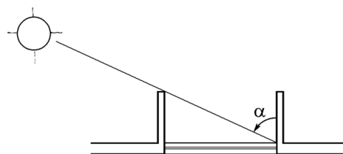
مقطع افقی - زاویه سایه بان عمودی
