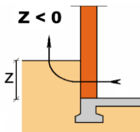
شکل پ ۱۱-۶ انتقال حرارت خطی دیوار مجاور خاک
