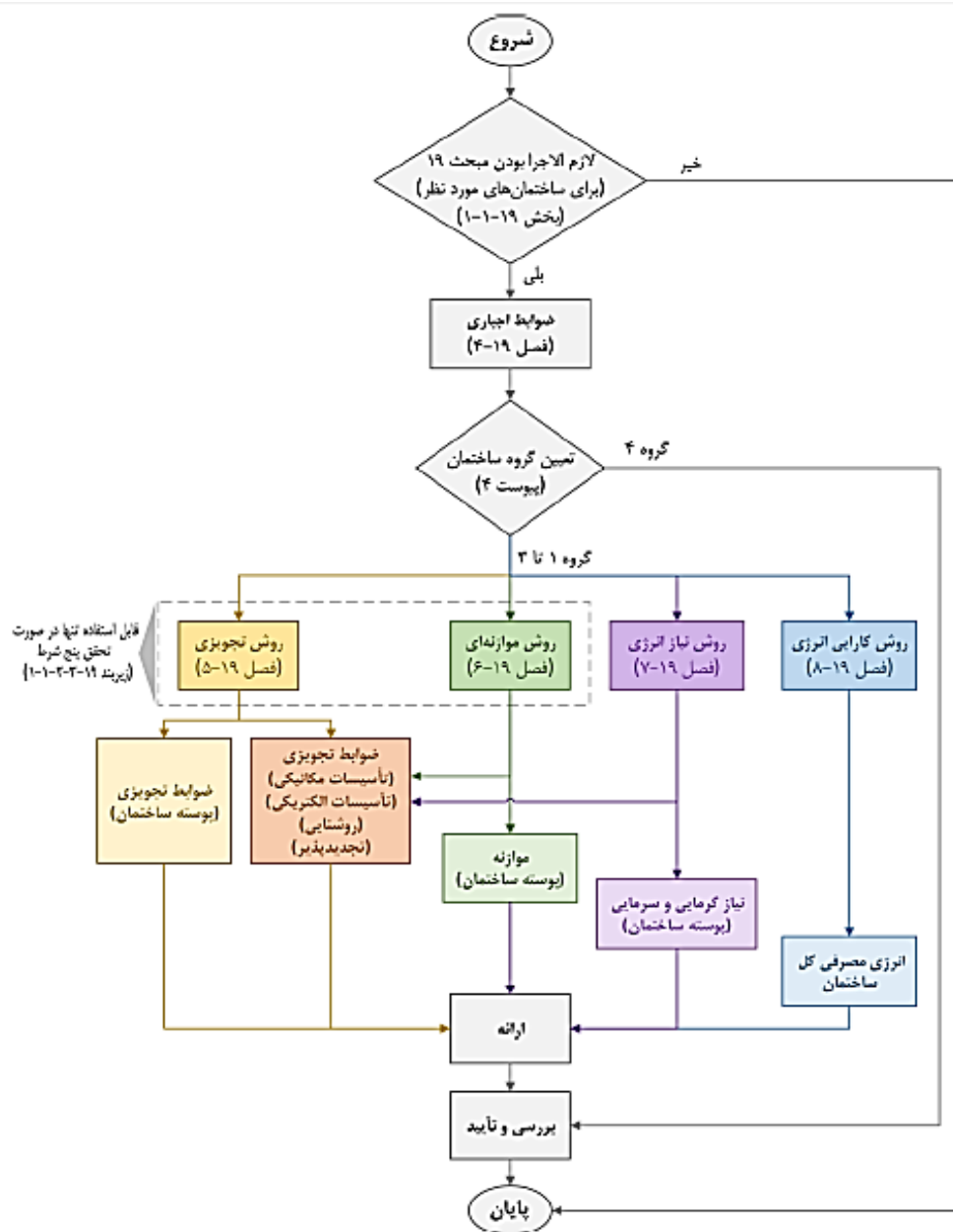
شکل ۱۹-۳ نمودار مراحل طراحی در چهار روش مختلف ارائه شده در این مبحث
