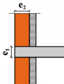
شکل پ ۱۱-۱۰ اتصالات متداول سقف‌های میانی
