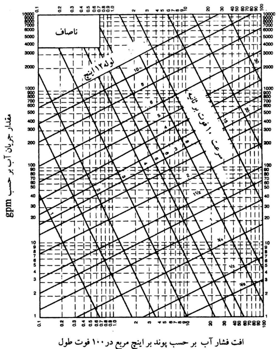
شکل پ ۱-۵-۴ (IP) اندازه گذاری لوله های فولادی گالوانیزه با سطح داخلی کاملاً ناصاف
