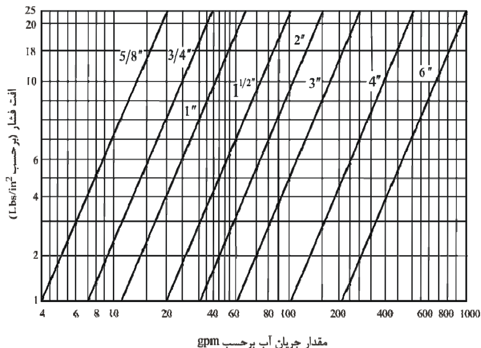
شکل پ ۱-۴-۲ (IP) - افت فشار در کنتور نوع دیسکی بر حسب پوند بر اینچ مربع
