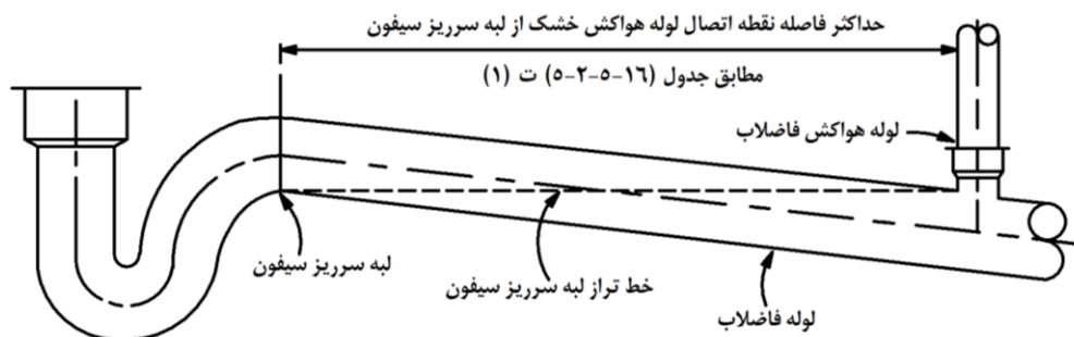
شکل ۵-۲-۵-۱۶ ت - اتصال لوله هواکش خشک لوازم بهداشتی
