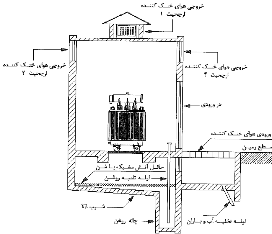
شکل ۵-۱۳-۳-۵-۱۳ (نوع الف) - طرحواره قائم اتاق ترانسفورماتور روغنی با تهویه طبیعی و هم‌سطح زمین
