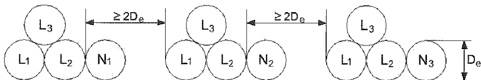
شکل ۱۳-۷-۱-۷-۱: آرایش مثلثی مخصوص برای ۹ رشته کابل تک رشته موازی (سه فاز)
