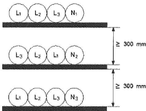
شکل ۱۳-۷-۱-۷-۱: آرایش چسبیده به هم در سه تراز و هر تراز به فاصله ۳۰ سانتی متر از هم برای ۹ رشته کابل تک رشته موازی (سه فاز)
