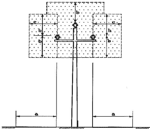
شکل پ ۱-۲-۷:۱ خط هوایی فشار متوسط (۱۱، ۲۰ و ۳۳ کیلوولت)
