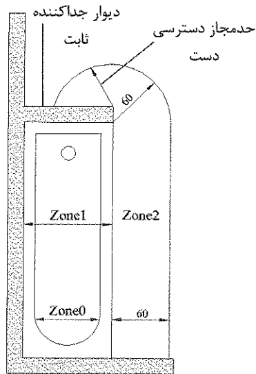
(۳) دید از بالا با دیوار جداکننده ثابت و خدمت‌جاز دسترسی دست
