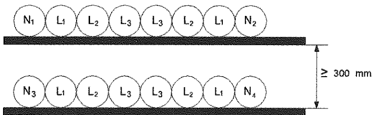
شکل ۱۳-۷-۱-۷-۱: آرایش چسبیده به هم در دو تراز به فاصله ۳۰ سانتی متر از هم برای ۱۲ رشته کابل تک رشته موازی (سه فاز)
