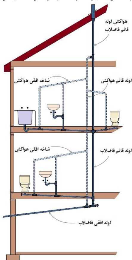
شکل (۳-۴): سیستم هواکش فاضلاب
