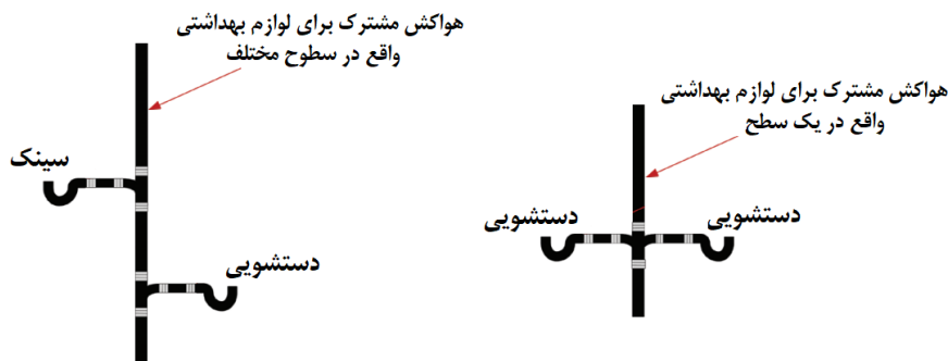
شکل (۳-۷): هواکش مشترک
