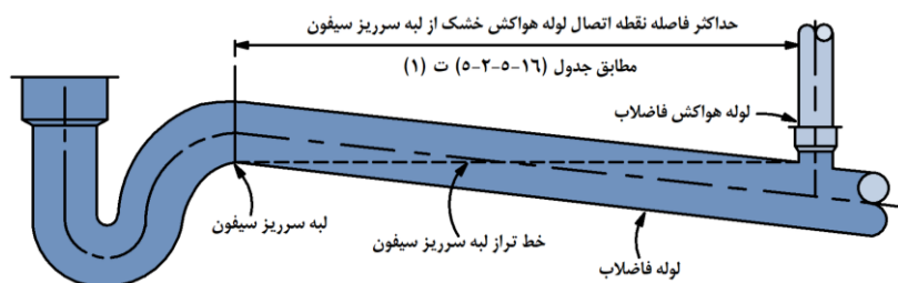
شکل (۳-۶): اتصال لوله هواکش خشک لوازم بهداشتی (طبق شکل ۱۶-۵-۲-۵ "ت")
